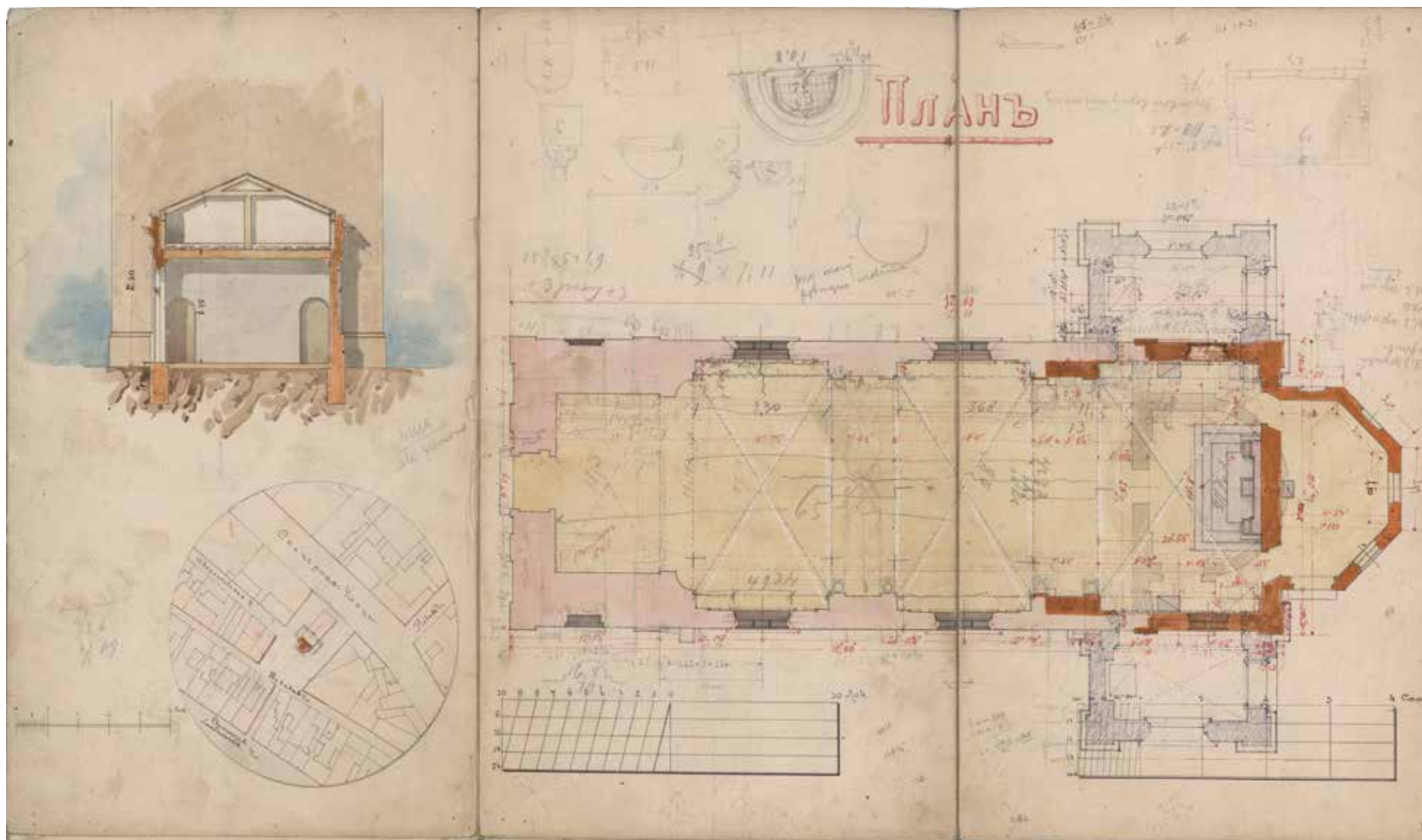
Projekt przebudowy Kościoła Ewangelicko-Augsburskiego w Radomiu, 1894 r.
