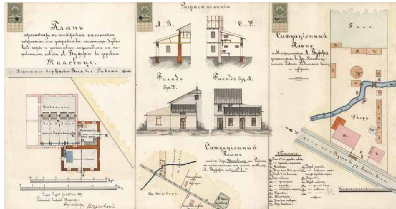
Plan budowy młyna kory dębowej i montażu maszyny parowej w garbarni ewangelika Ludwika Buffa we wsi Żakowice, 1909 r.
