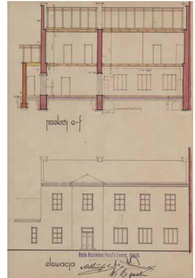
Projekt urządzenia świetlicy w domu Parafii Ewangelicko-Augsburskiej w Radomiu autorstwa inż. Alfonsa Pinno (fragmenty), 1939 r.
